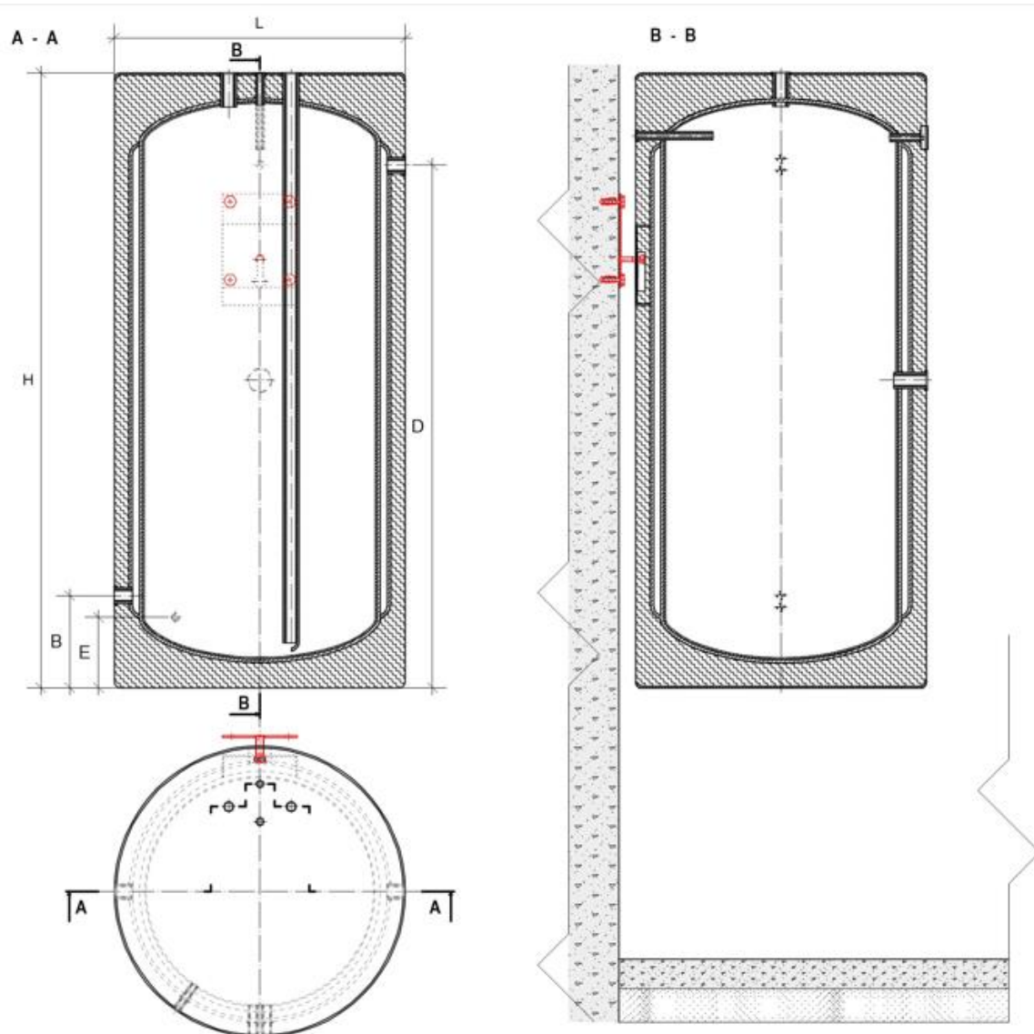
RYS. TECHNICZNY
