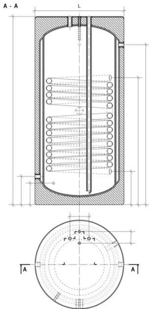
RYS. TECHNICZNY
