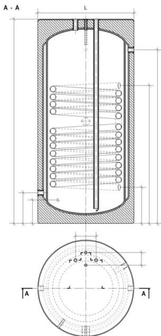
RYS. TECHNICZNY
