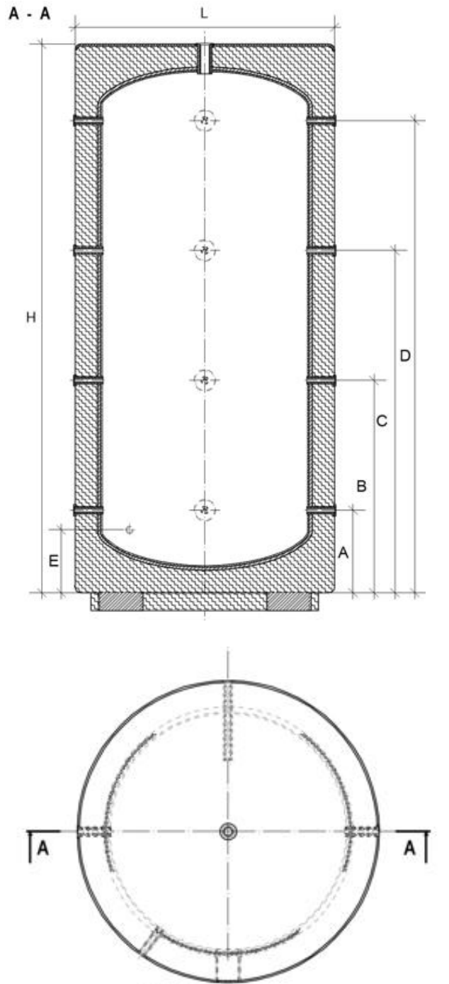
RYS. TECHNICZNY
